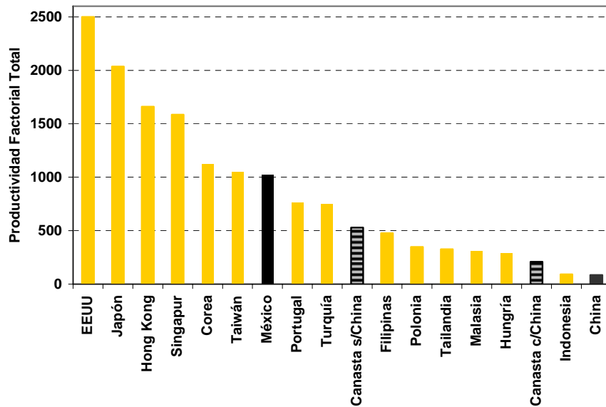
(b) PFT
